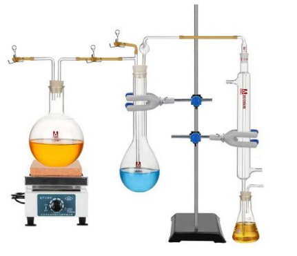
煤中氮测定装置
